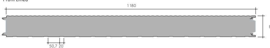
Profil Twinlook
