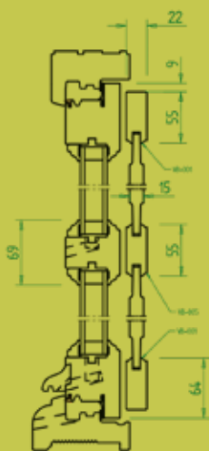
COUPE VERTICALE
