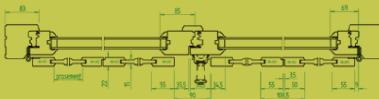
COUPE HORIZONTALE
