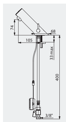
Mitigeur TEMPOMATIC 5 avec pile Réf. DELABIE : 499006
