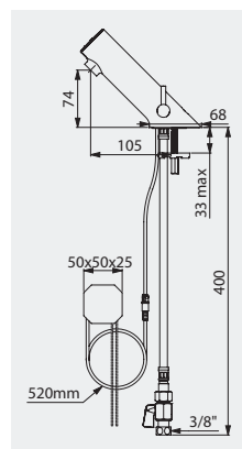
Mitigeur TEMPOMATIC 5 sur secteur Réf. DELABIE : 499000
