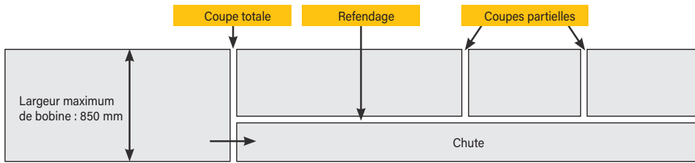
Coupe partielle avec élimination de la chute
