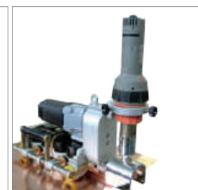
Modèle présenté Réf. SER100A-05WAD avec l'option SER-05SETHIVER
