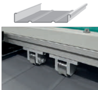
Galets de nervurage en fond de bac Réf. PROBAC-HT-NERV
