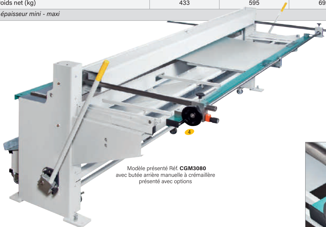
Réglage de la butée arrière par volant
