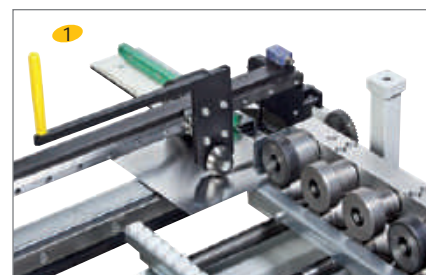
1 Coupe transversale manuelle
