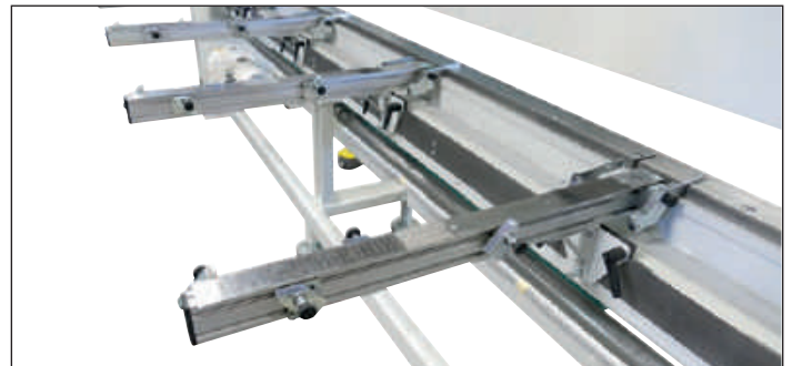
Butée arrière manuelle à glissière, course maxi 750 mm Réf. PTL-BAM
