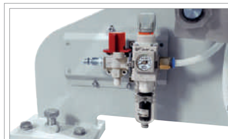
L'assistance pneumatique nécessite un branchement en air comprimé: débit minimum 200 litres/minute, 8 bars minimum (compresseur non fourni)
