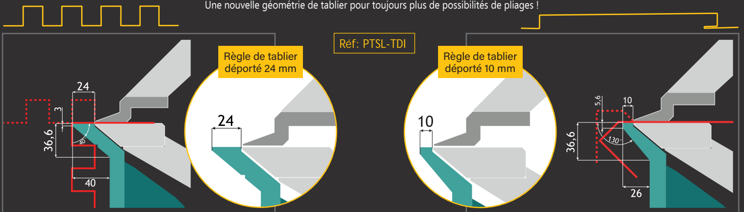
Pliages en créneaux / omégas
