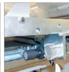
2 Système pneumatique pour la conicité de la butée arrière
