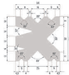
Bloc multi-vé livré avec presse plieuse de 30 et 50 tonnes
