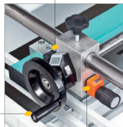
Réglage de conicité de la butée
