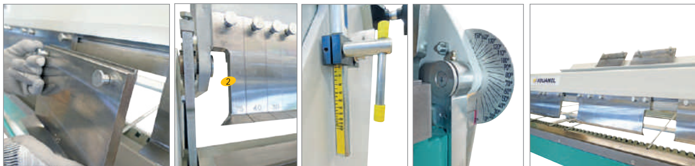
1 Démontage rapide des segments par tirette
