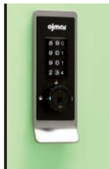
550.015 - Serrure COMBI à combinaison mécanique - Utilisable en code fixe ou en code libre - déverrouillage d'urgence par clé passe-partout
