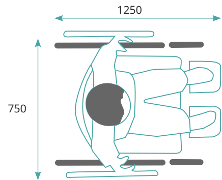
Dimensions usuellement prises en compte pour un fauteuil roulant
