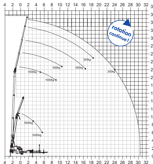
Double vérins de jib
