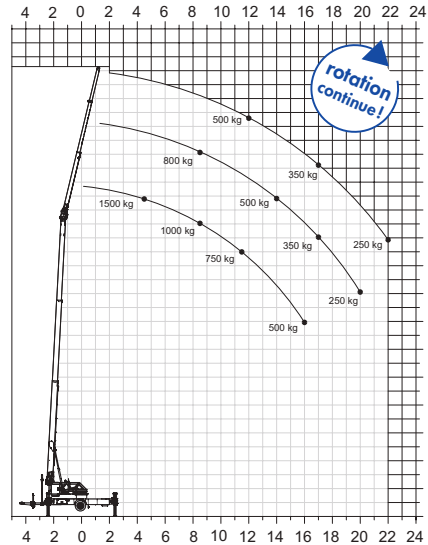
Jib télescopique hydraulique
