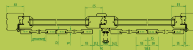
COUPE HORIZONTALE
