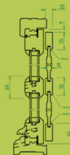
COUPE VERTICALE
